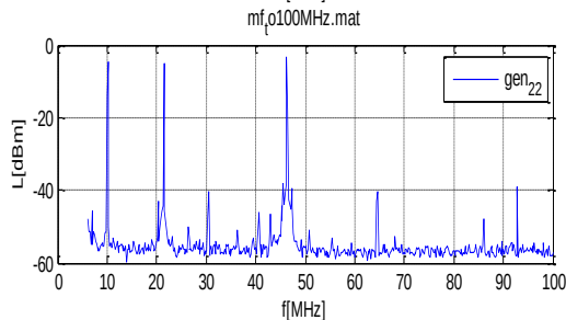
Náhled spektra generovaného signálu
