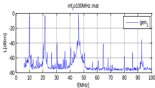
Sestavený generátor
