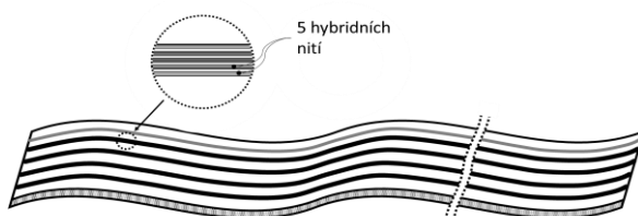
Topologie pružné vodivé stuhy ve čtyřvodičovém provedení.
