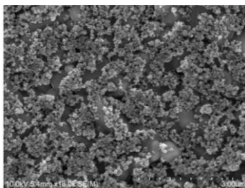
Obr. 2: SEM snímek senzitivní vrstvy SWCNT/ \text{In}_x\text{O}_x / \text{SnO}_x s platinovými nanočásticemi (Pt NPs).
