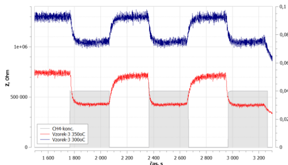
Obr. 4: Odezva senzorů na skokovou změnu koncentrace \text{CH}_4 (0,04 %) při teplotě 300 °C a 350 °C.
