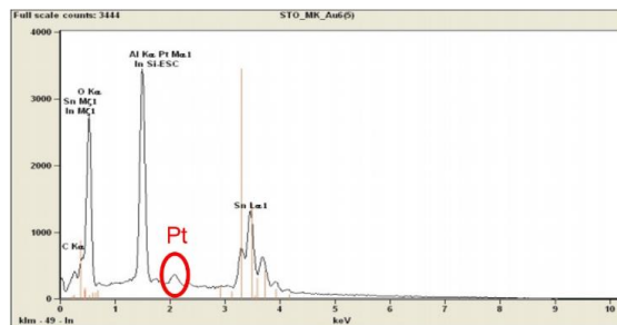
Obr. 3: EDX analýza senzitivní vrstvy SWCNT/ \text{In}_x\text{O}_x / \text{SnO}_x s platinovými nanočásticemi (Pt NPs).
