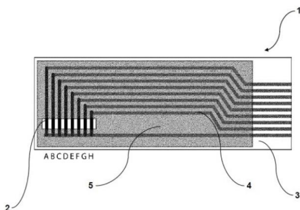
Obr. 1: Uspořádání tištěného senzoru obsahujícího natištěné senzorové elementy A–H, které reagují na různé typy kapalin.
