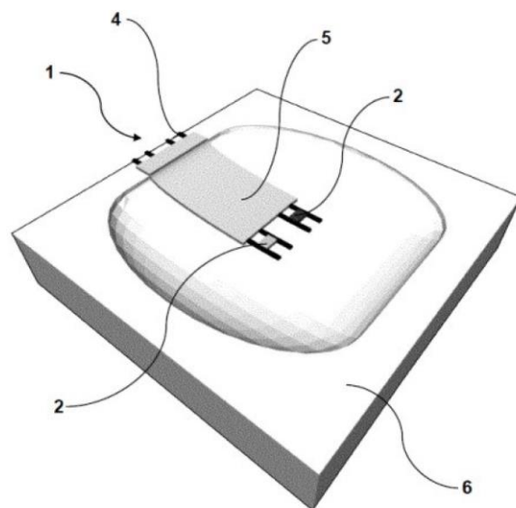
Obr. 2: Elektronický senzor se dvěma senzorovými elementy natištěný na 3D povrchu.
