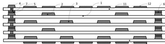
Schématické znázornění technologického provedení vyvinutého senzoru v bočním řezu
